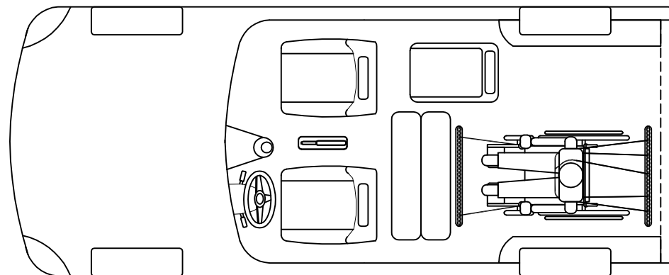
CONFIGURAZIONE CON N° 3 POSTI SEDILE COMPRESO CONDUCENTE + UNA SEDIA A ROTELLE
