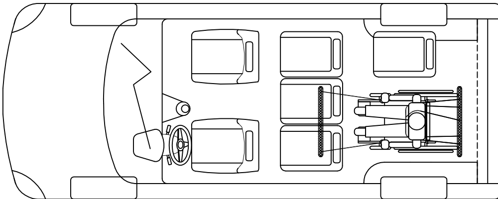
CONFIGURAZIONE CON N° 6 POSTI SEDILE COMPRESO CONDUCENTE + UNA SEDIA A ROTELLE
